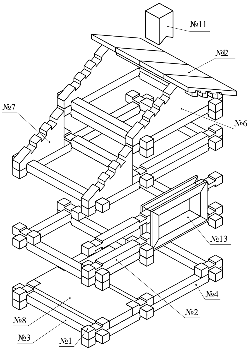
Последовательность сборки домика
