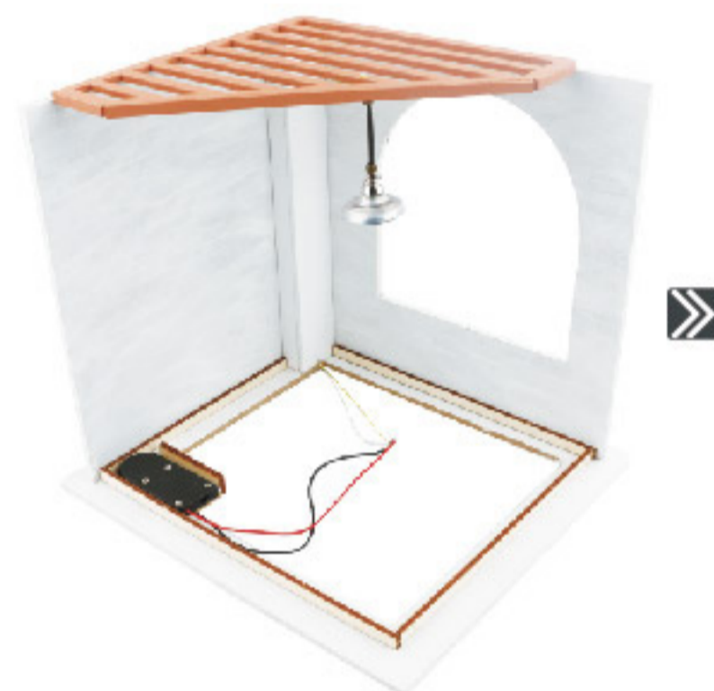
17 Соедините провода из диода с проводами из блока питания. Соедините красный провод с желтым и белый с черным. Проверьте, работает ли лампа.
