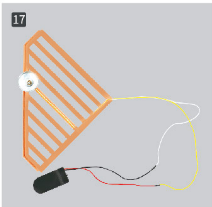
17 Соедините провода из диода с проводами из блока питания. Соедините красный провод с желтым и белый с черным. Проверьте, работает ли лампа.
