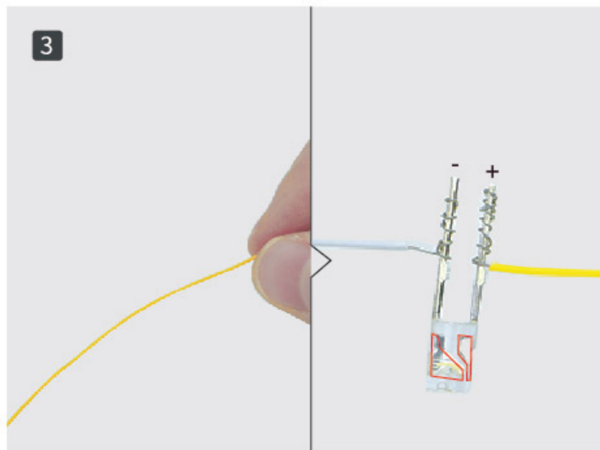
3 Зачистите по 12 мм с желтого и белого проводов и соедините их с диодом. Обратите внимание на полярность.
