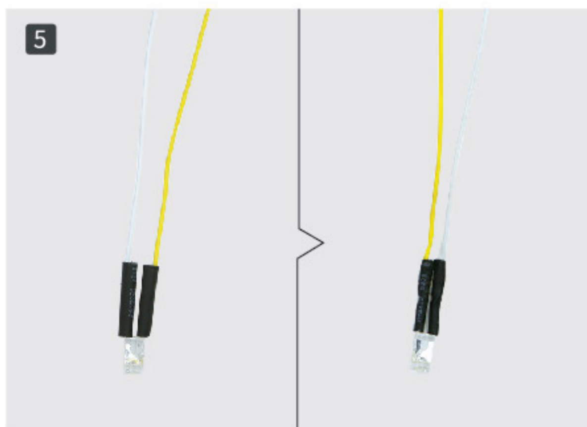
5 Отрежьте 2 6-миллиметровых куска термоусадочной трубки и пропустите через них провода, как на иллюстрации. Используйте зажигалку, чтобы быстро нагреть термоусадочную трубку для изоляции проводов.
