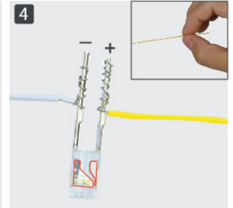
4 Снимите по 12 мм изоляции проводов. Присоедините диод, как показано на иллюстрации.
