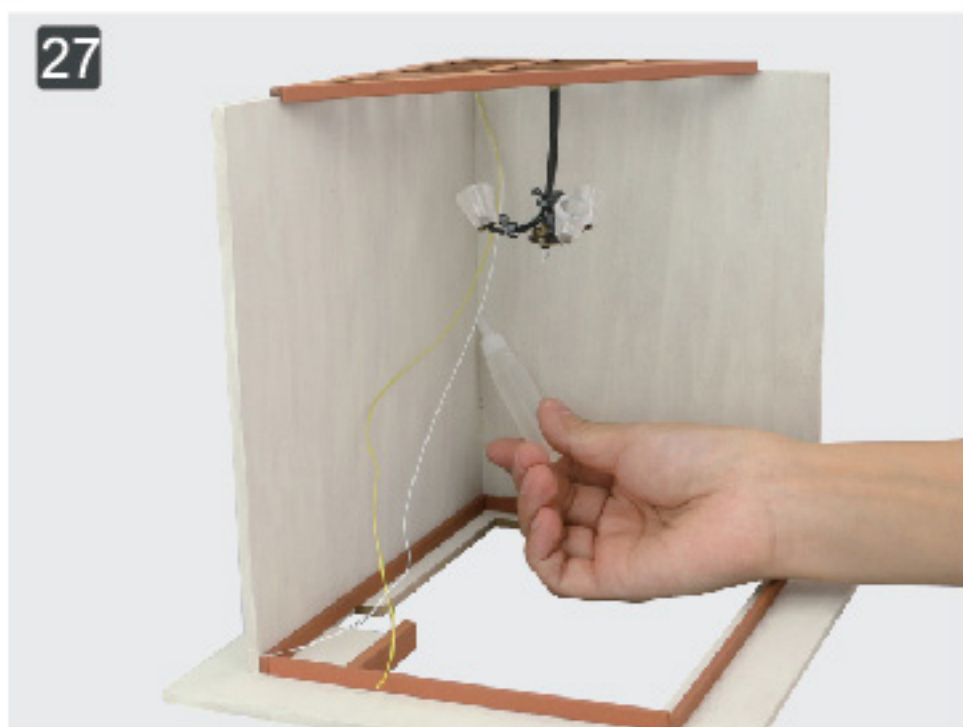
27 Приклейте провод к стене. Не приклеивайте (B1) к стене.
