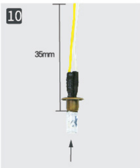
10 Повторите шаги 3–5, обрежьте до 35 мм.
