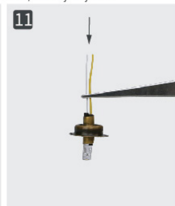
11 Пропустите сквозь отверстие и металлическую накладку.
