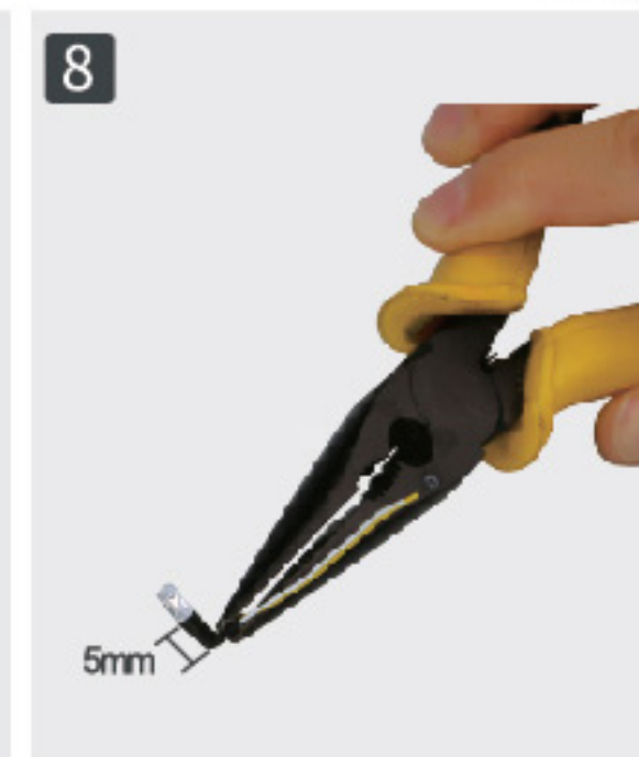
8 Согните, как на иллюстрации.
