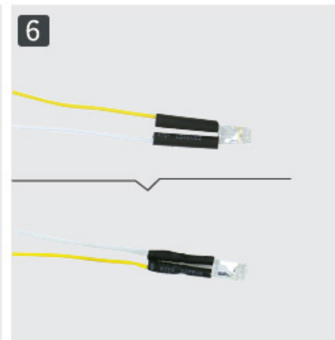
6 Разрежьте утягивающуюся трубку на 10 мм, всего 2 шт. Проденьте провода в трубку. Подогрейте трубку с помощью огня, чтобы утянуть её.
