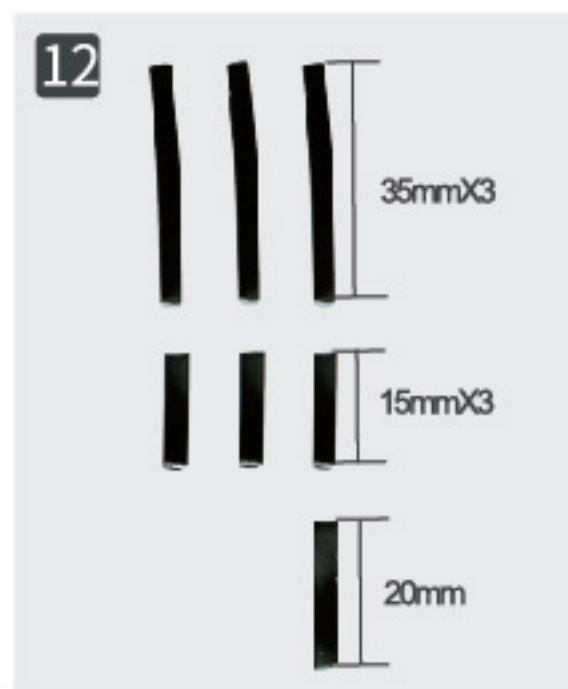
12 Обрежьте, как на иллюстрации.
